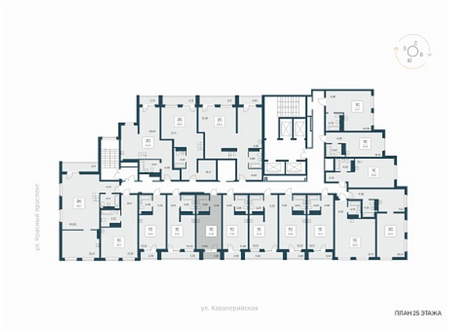
План этажа
